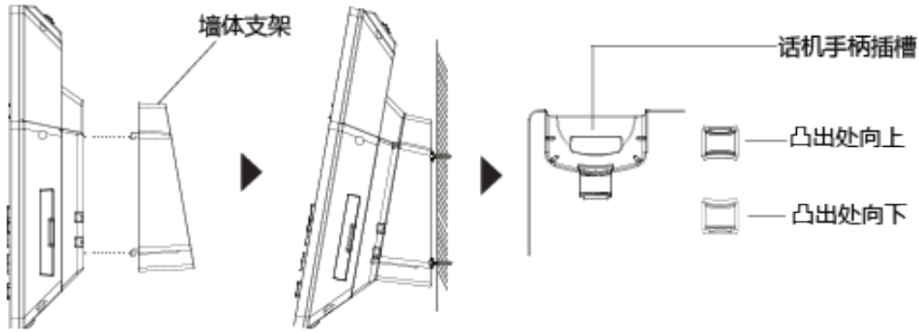
图 3: 手柄插销
