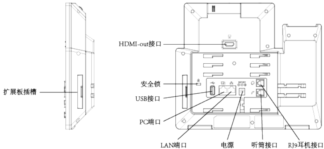
图 4: GXV3350 背面/侧面图
